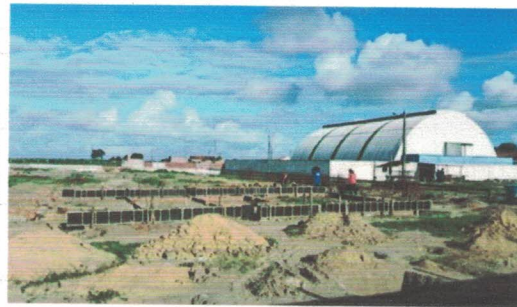
Execução das vigas baldrame, montagem de formas (-9.7709817, -36.3474868) Data: 07/05/2026
