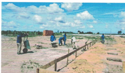
Escavação e concretagem das bases (-9.7709817, -36.3474868) Data: 09/04/2026
